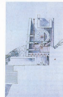
Cyclopentoren, doorsnede.
