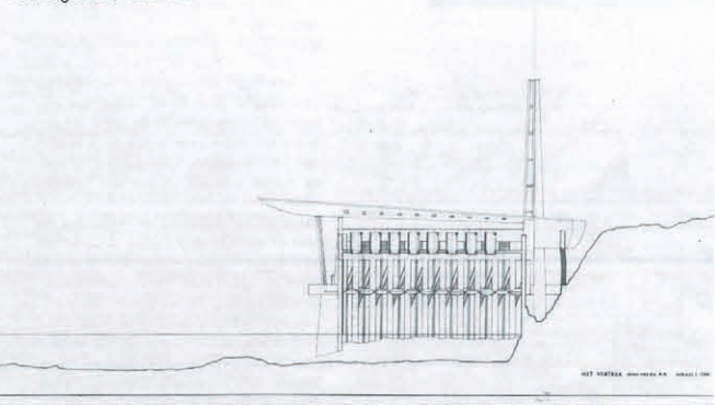
Vertrekgebouw, doorsnede.
